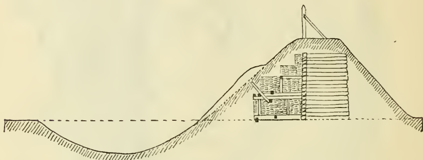
Fig. 127. — Constructions en bois de la chaussée de Bělgorodka.
