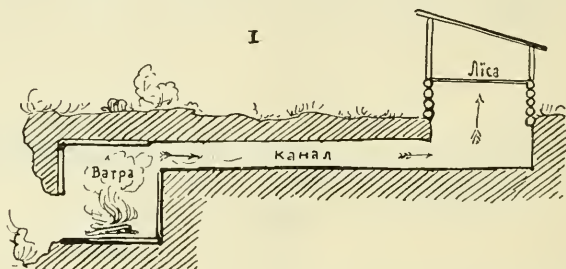
Fig. 41. — Coupe d'un séchoir (ватра « feu », ліса « soupente en claies »).
