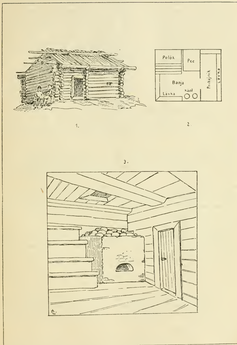
Fig. 1. — Bain russe du gouvernement de Novgorod le Grand ( banja « chambre du bain », pribajnik « antichambre », polok « estrade en bois », pec « poêle », lávka « banc »).
