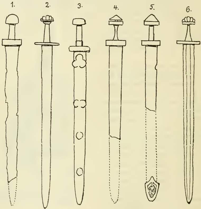
Fig. 105. — Épées slaves (1. Hohenberg ; 2. Koljany ; 3. Jarohňovice, 4. Kiev ; 5. Gnězdovo ; 6. Golcow).
