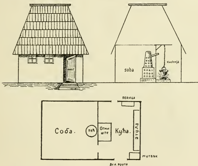
Fig. 39. — Maison serbe ( kuća ) de Bosnie. ( soba « chambre à poêle », kuhna « cuisine à foyer »).
