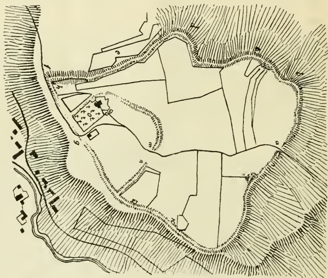
Fig. 125. — Plan du hradiště de Budeč, en Bohême (type à un seul faubourg).
