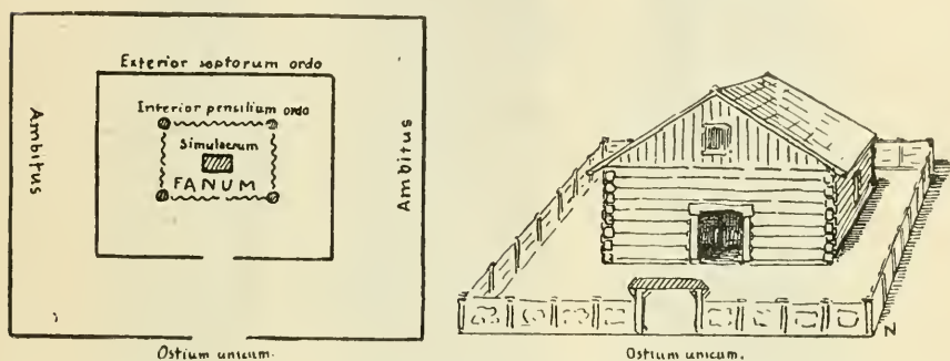
Fig. 50. — Plan et reconstitution du temple de Svantovit à Arcona.
