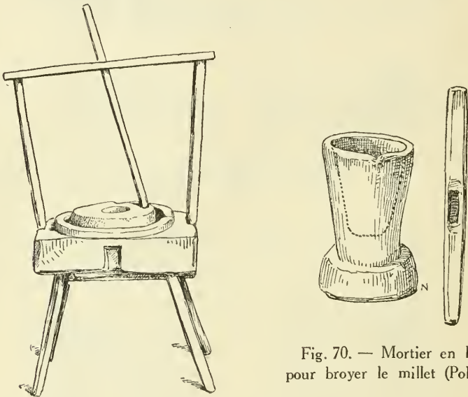
Fig. 69. — Ancien moulin tchèque. (Musée d'ethnographie de Prague).
