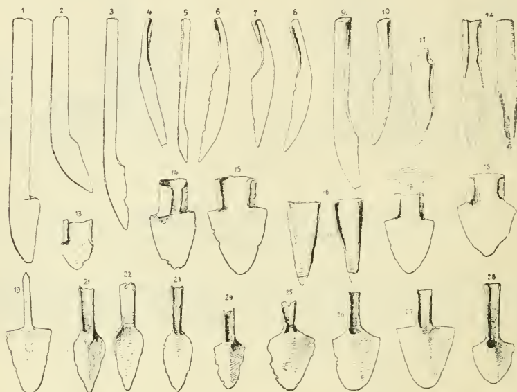
Fig. 61. — Coultres et socs romains des musées de Zagreb, Ljubljana et Sarajevo.
