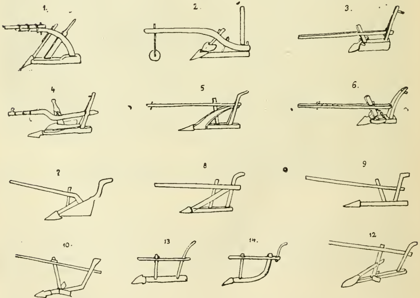
Fig. 57. — Araires slaves au bois glissant.
